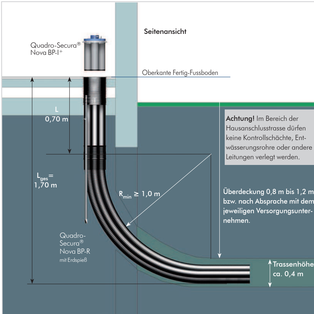
Abb. 7: Einbau Quadro-Secura® Nova BP+
